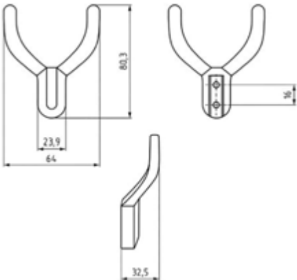
КРЮЧОК МЕБЕЛЬНЫЙ FHK-19803
