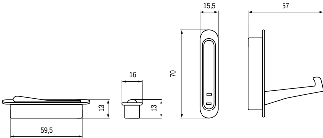
КРЮЧОК МЕБЕЛЬНЫЙ FHK-14903
