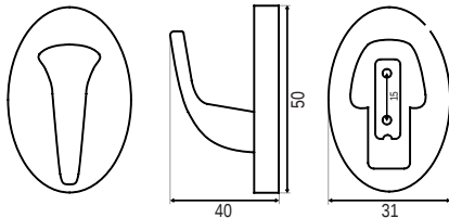
КРЮЧОК МЕБЕЛЬНЫЙ FHK-15303
