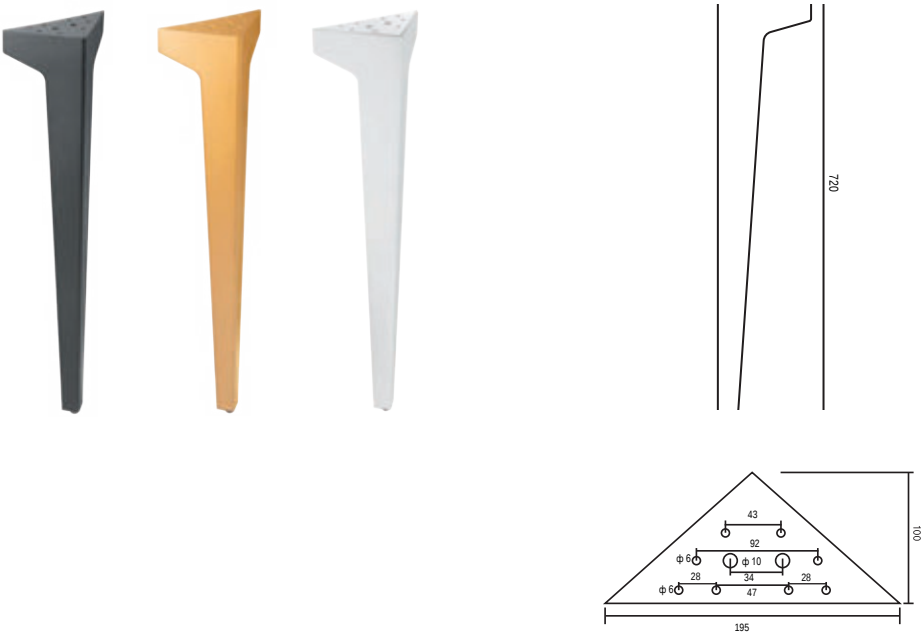
ОПОРА ДЛЯ СТОЛА 720*135
