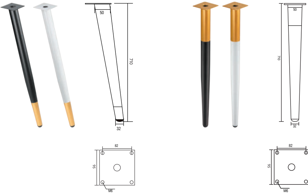
ОПОРА ДЛЯ СТОЛА 710*50
